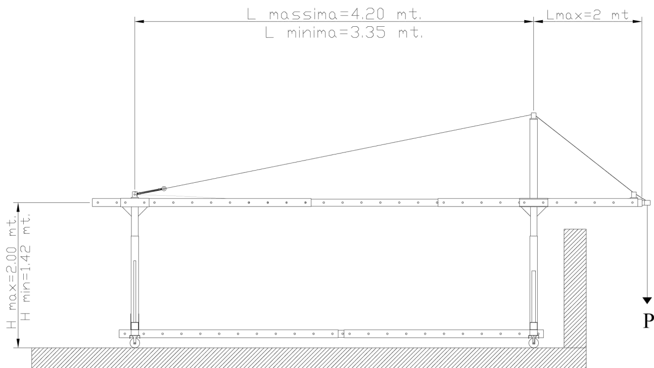
SCHEMA SOSPENSIONE SEMPLICE
